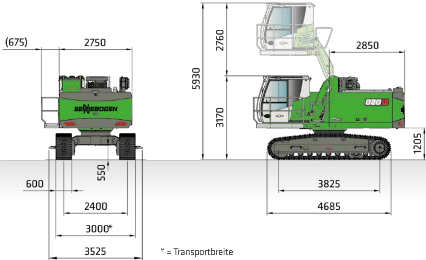
828 G MIT RAUPENUNTERWAGEN R35/240 UND HYDRAULISCH HOCHFABRBARER KABINE G280 (SERIE)
