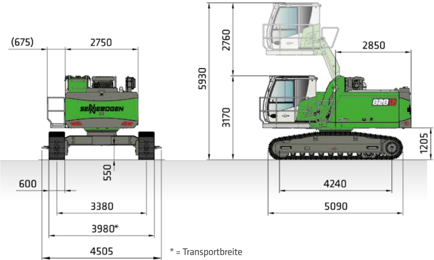
828 G MIT RAUPENUNTERWAGEN R35/340 UND HYDRAULISCH HOCHFABRBARER KABINE G280 (SERIE)
