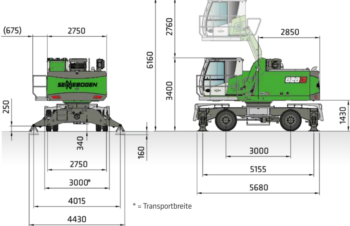
828 G MIT MOBILUNTERWAGEN MP27 UND HYDRAULISCH HOCHFABRBARER KABINE G280 (SERIE), VOLLGUMMI-BEREIFT 10.00-20 (8-FACH)
