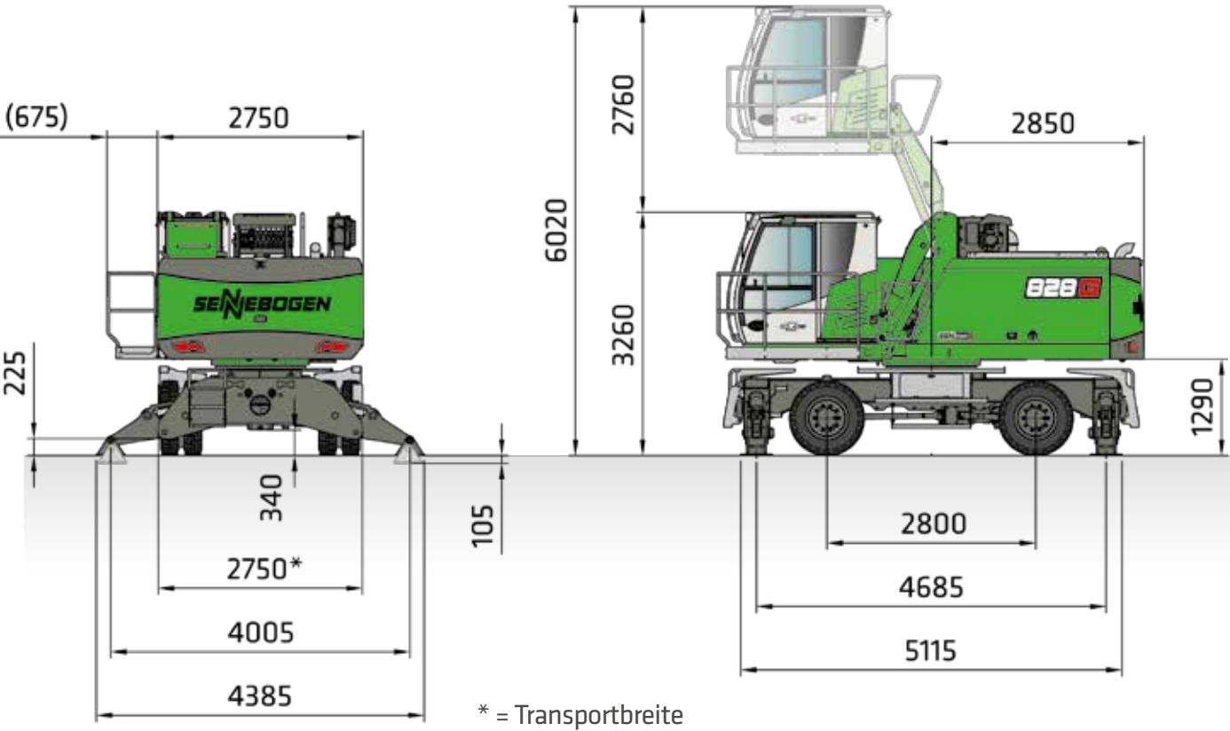
828 G MIT MOBILUNTERWAGEN MP26 UND HYDRAULISCH HOCHFABRBARER KABINE G280 (SERIE), VOLLGUMMI-BEREIFT 10.00-20 (8-FACH)
